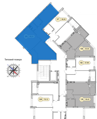
План типового поверху
